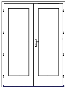
Nr. 42 Double door 58 mm DG 1425 x 1955 mm R
