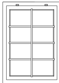
Fenster 40 mm 865 x 1210 mm 2 stk.
