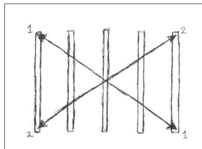
Fig. 2. Diagonalmål: Skal give samme mål på længde 1 og 2.
