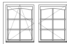
NR. 020 Doppelfenster ISO 58 mm 1530 x 990 mm 1 st.
