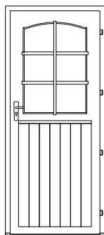
NR. 19-1 Einzeltür ISO 58 mm 840 x 1955 mm 1 st.
