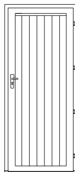
NR. 19-2 Einzeltür 58 mm 840 x 1955 mm 1 st.
